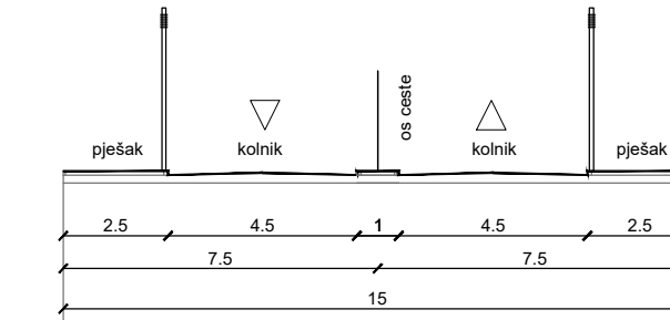
KARAKTERISTIČAN POPREČNI PRESJEK B-B
