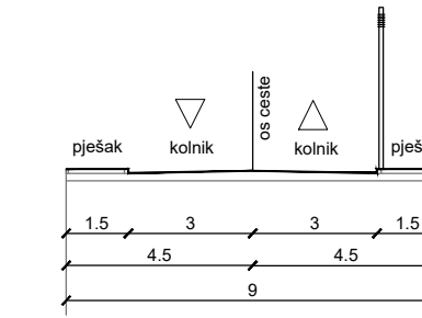
KARAKTERISTIČAN POPREČNI PRESJEK C - C
